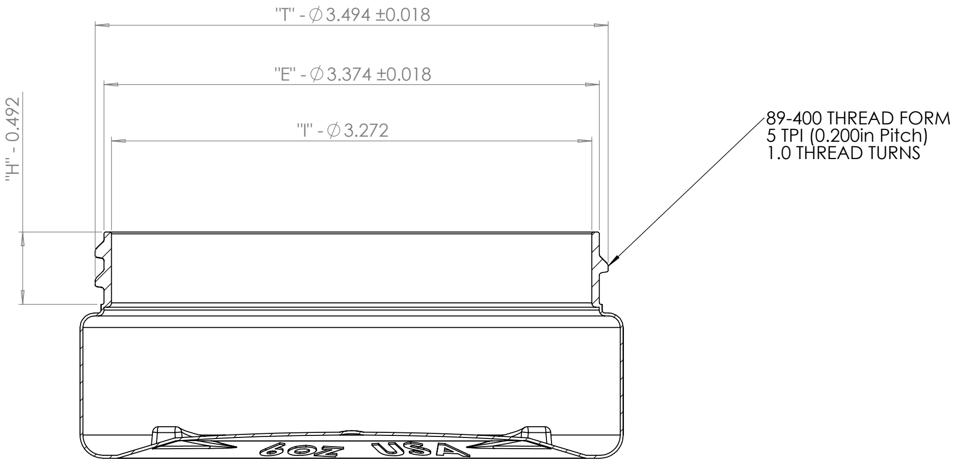
SECTION A-A
